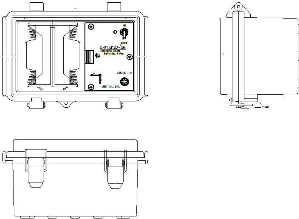
装置本体概略図
